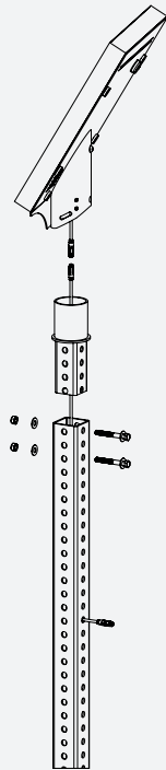
2" Telespar
